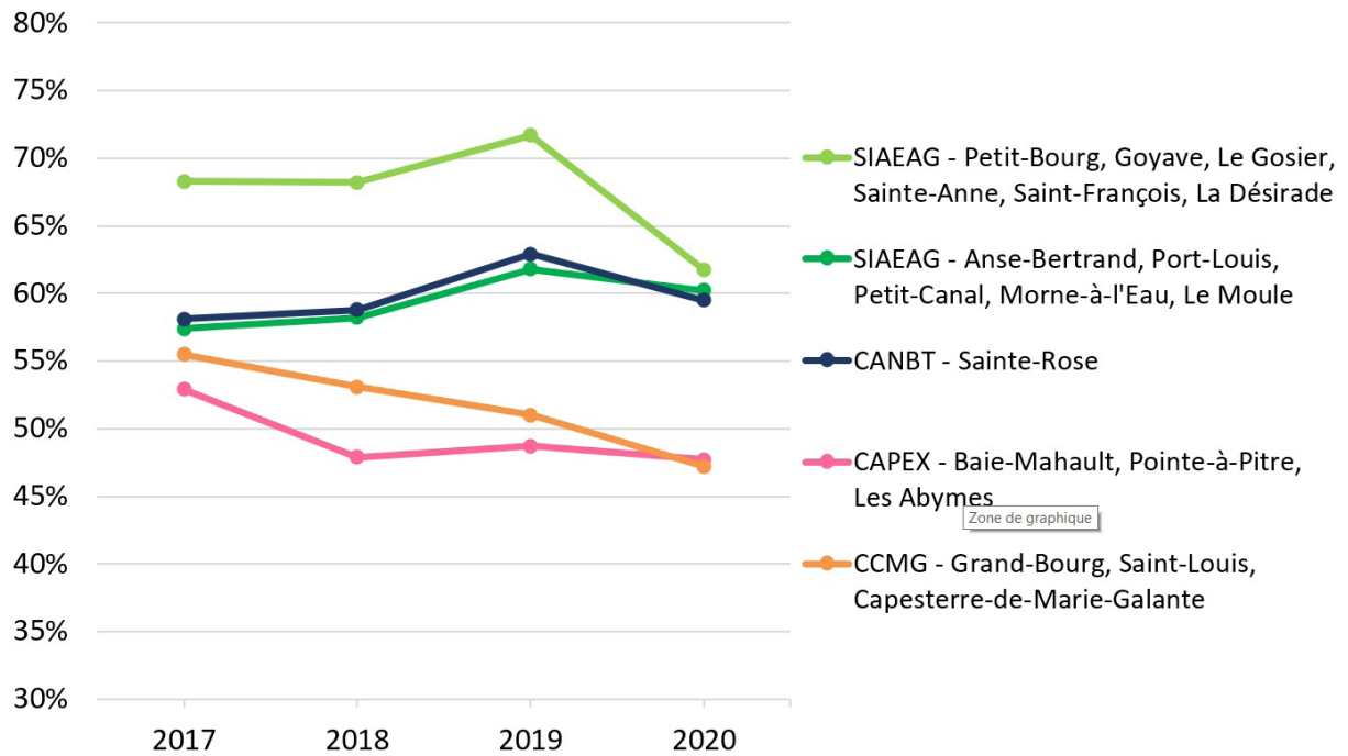
Figure 33 : Évolution annuelle des taux de pertes sur les territoires présentant une amélioration de la situation entre 2019 et 2020 (source : SISPEA)
