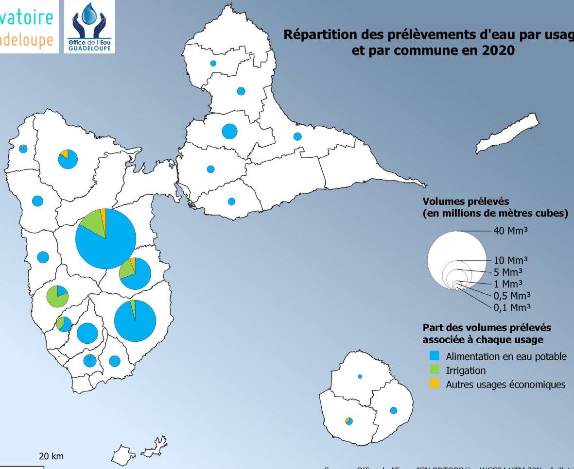
Figure 16 : Répartition des prélèvements d'eau par usage et par commune en 2020 (source : Office de l'Eau)
